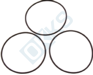
►15202 XXX27-1 Ø 109.22 mm
