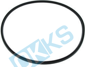
370 KÜLBÜLATÖR KAPAK LASTİĞİ BÜYÜK-ESKİ MODEL Cylinder Ring Rubber 111996030 370 x 329 x 3,50 MM
